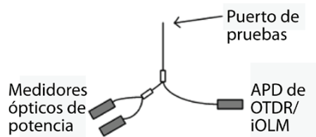
Ilustración 5-4. Medidor de potencia en línea
