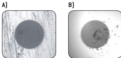
Ilustración 3-3. a) Arañazo en la región del núcleo b) Despostillado en el revestimiento
