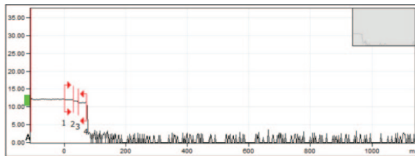
Ilustración 3-13. Curva OTDR utilizando una amplitud de pulso corta
