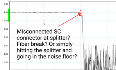
그림 2. Last-mile OTDR 트레이스.
