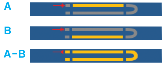
iOLM에서 루프백 테스트 방식과 iLOOP 옵션을 사용하면 파이버 두 개를 한꺼번에 테스트할 수 있습니다. A 링크만, B 링크만 보거나 루프까지 포함해 A-B 링크 전체를 볼 수 있습니다.
