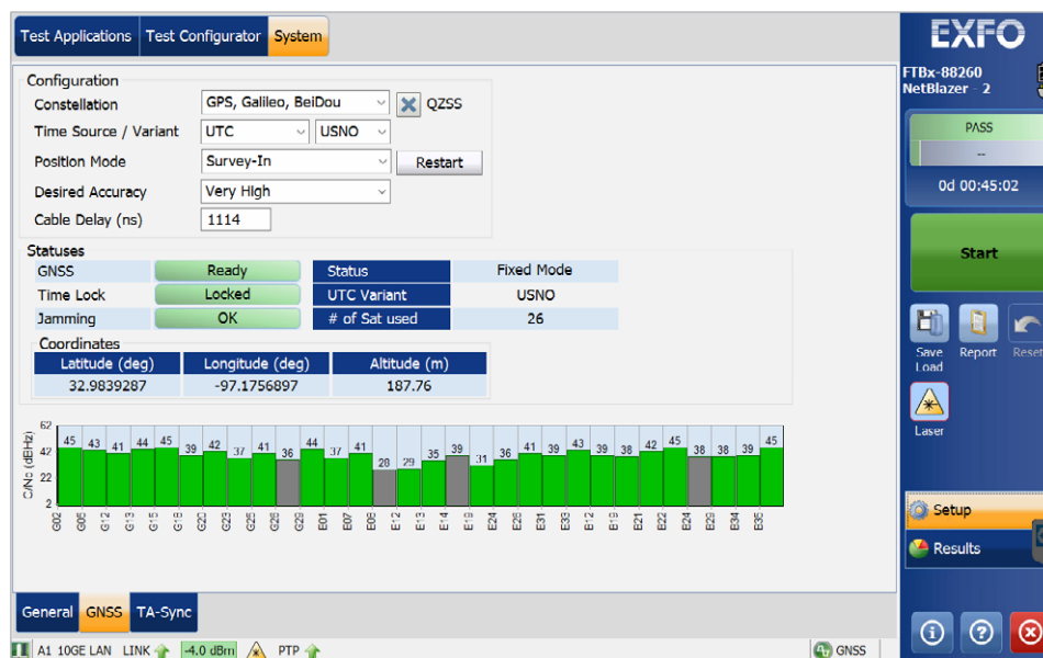
图5: 集成的GNSS配置和状态用户界面。
